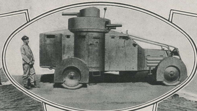
AUTOMOBILE BLINDÉE ANSALDO EN ORDRE DE MARCHÉ
