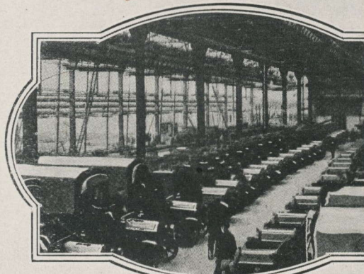
BATTERIES DE 102-35 SUR AUTOS-CAMIONS
