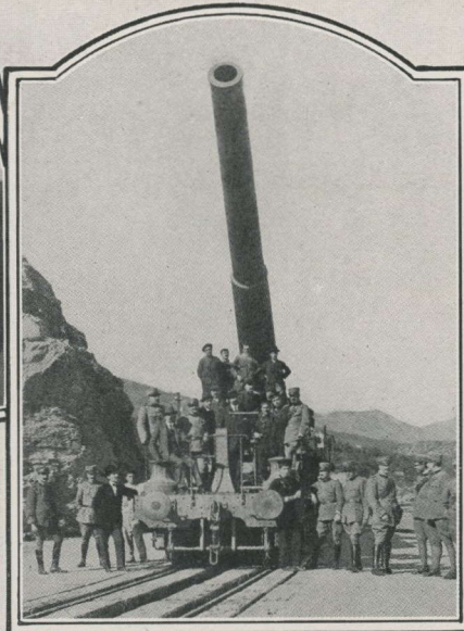
CANON DE 885 SUR AFFUT-TRAIN
